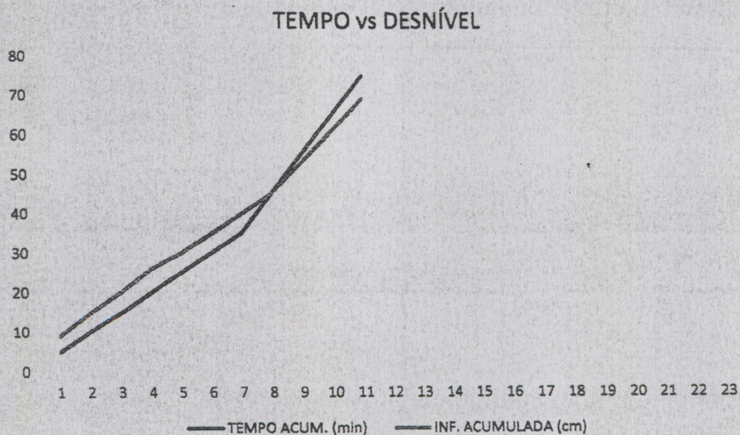
Gráfico 02 – Gráfico do ensaio PT 02.
